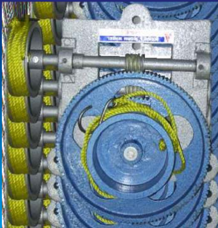
Worm & Wirm Wheel
