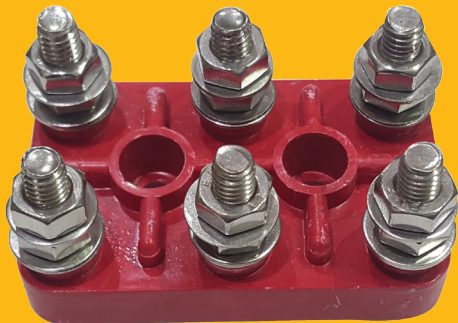
EF 5-6 ABB 15 HP DMC SS
