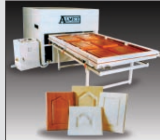
Membrane Press
